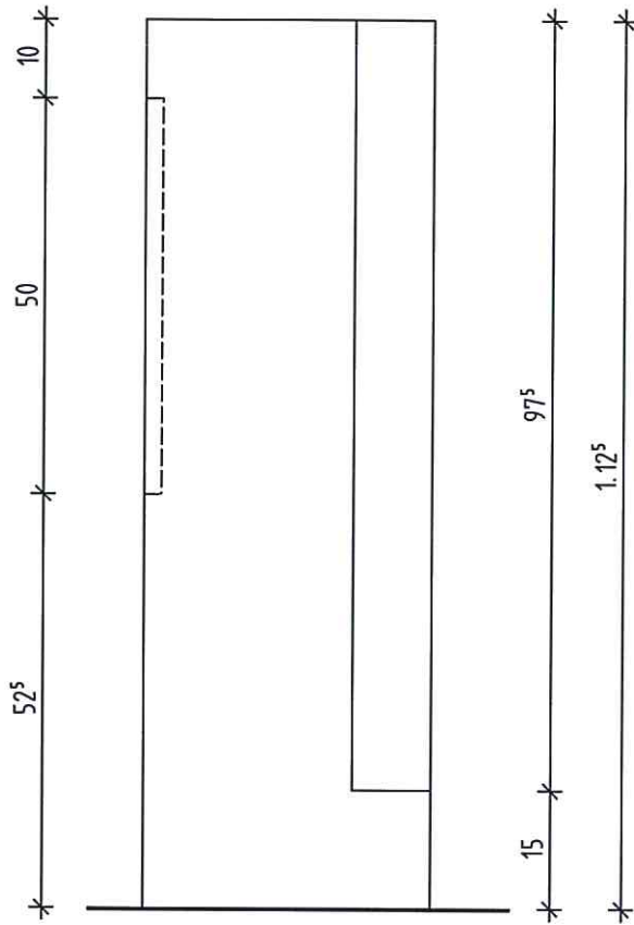
Ansicht
