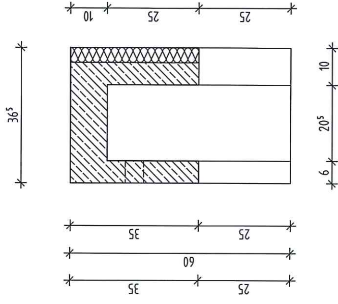
Schnitt A - A'
