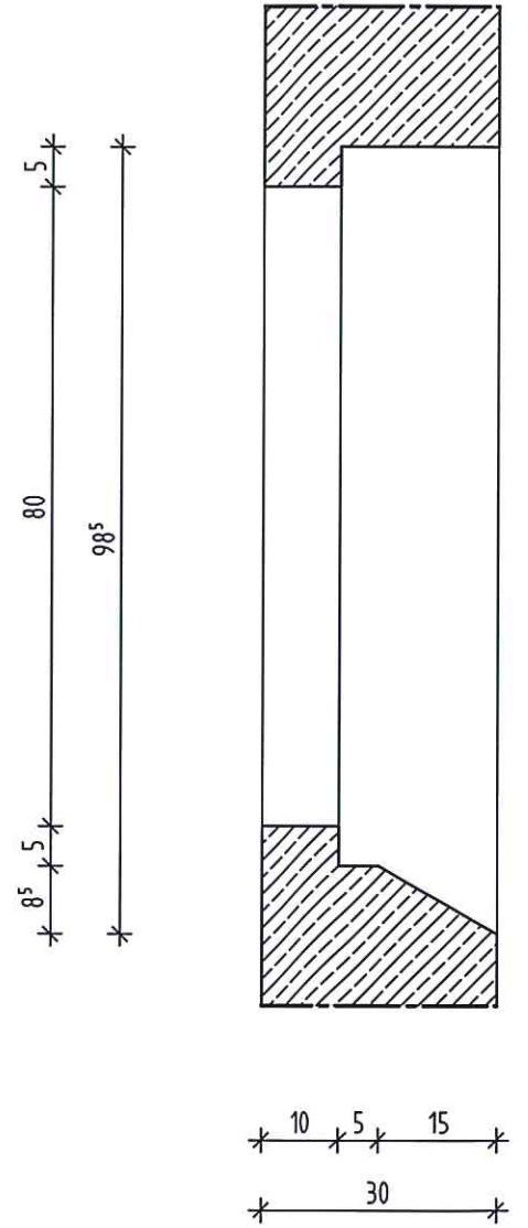
Schnitt B - B'
