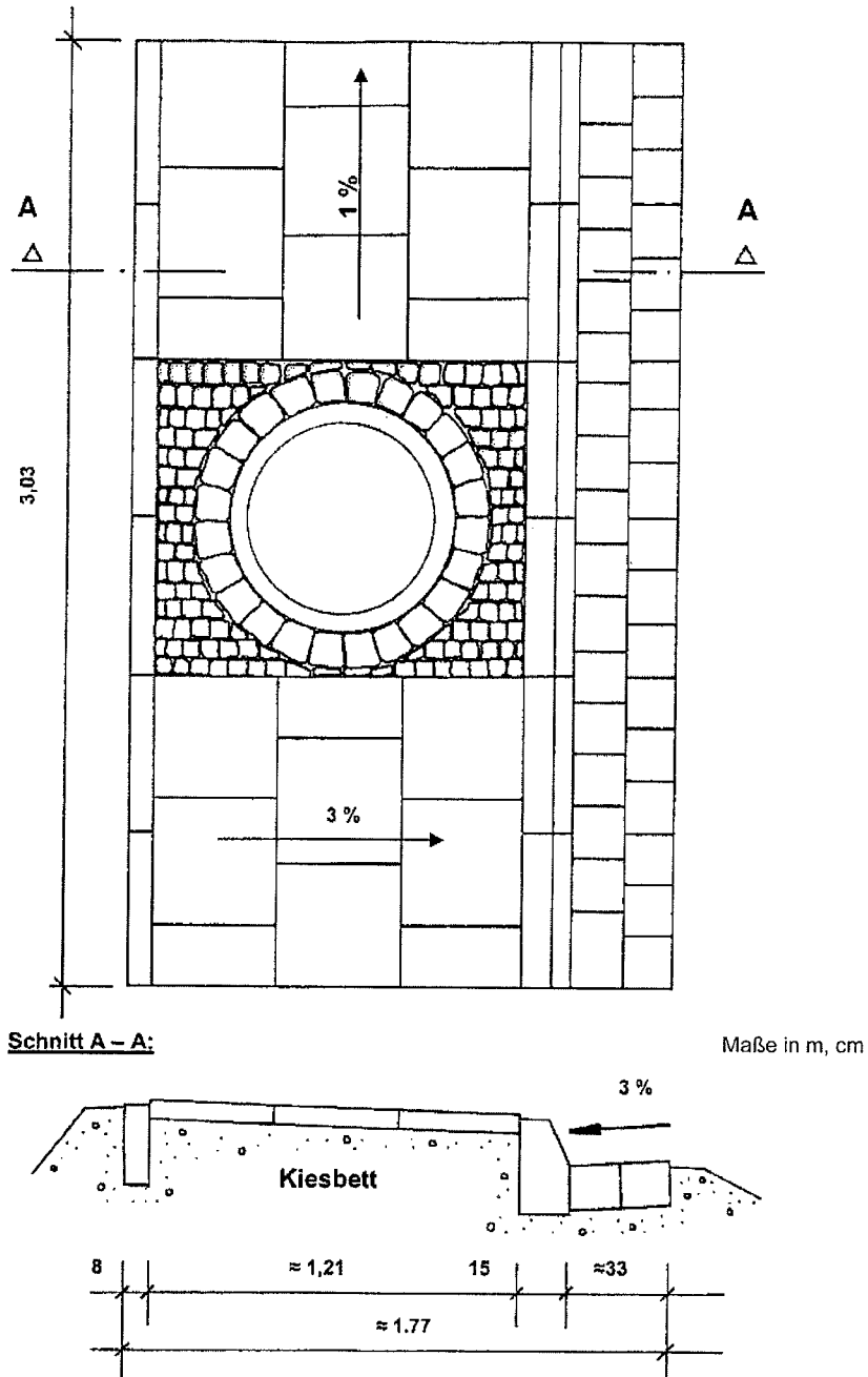
Abb.: 7 - 1 Abmessungen des Gehweges
